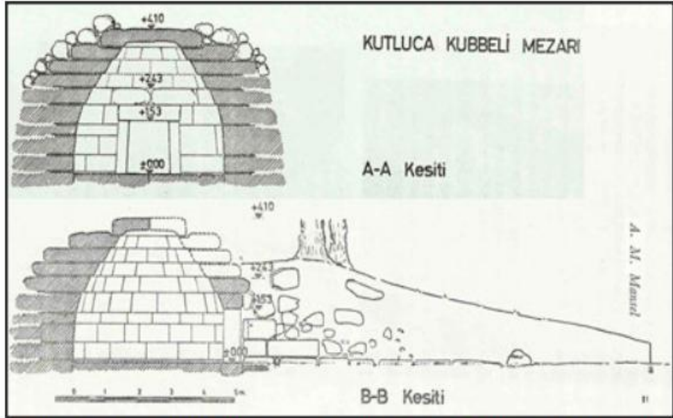
Çizim 2: Kutluca Tümülüsü mezar binası kesitleri (Mansel 1973, Res. 10).
