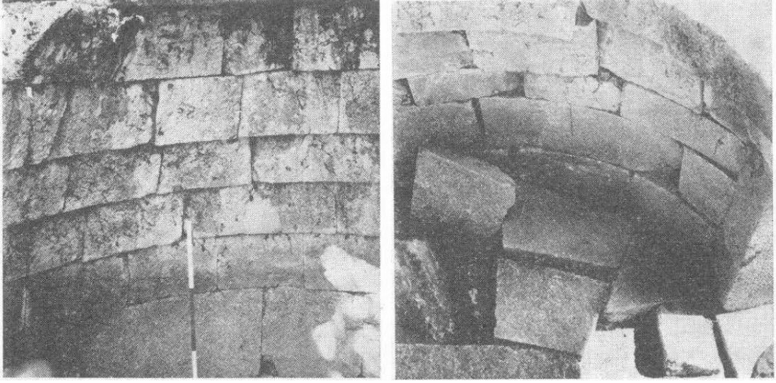
Şekil 15: Kutluca Tümülüsü - Kubbe İçi (Mansel, 1968: s. 109, Resim. 5-6)
